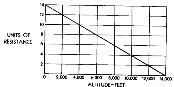
FIG. 11 ALTITUDE COMPENSATOR
